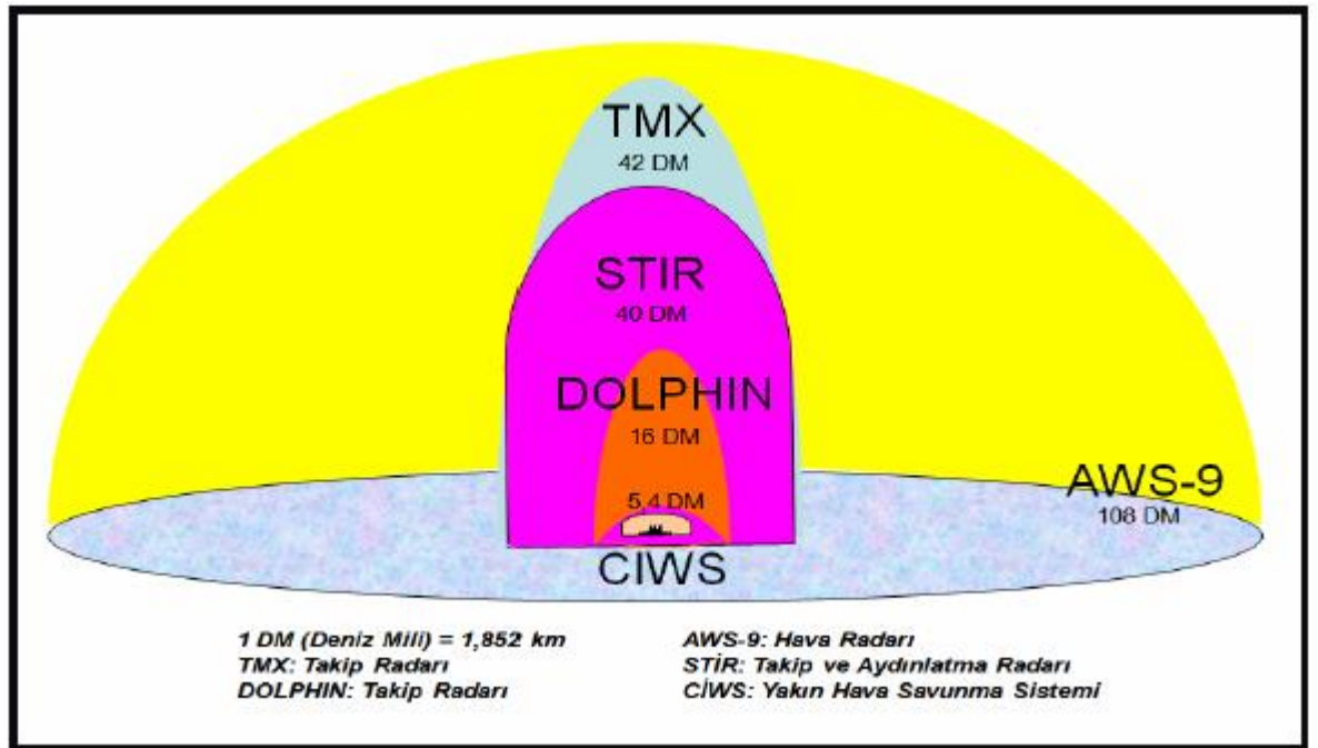
Şekil 22: MEKO Sınıfı Fırkateyn Sensör Kaplama Alanlar (Günümüz Muharebelerinde Ateş Desteğinin Önemi, 2015: 58)
