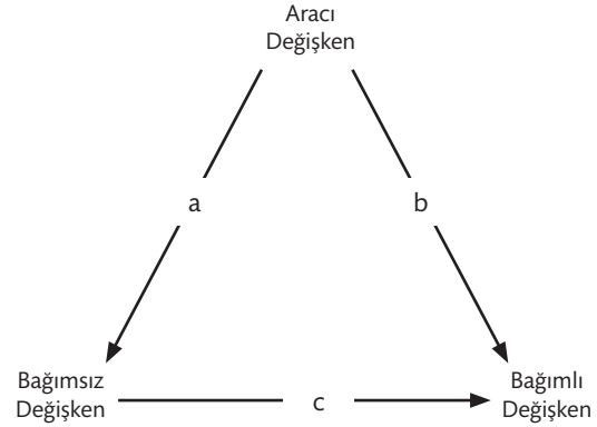
Şekil 1. Aracı etki modeli.
