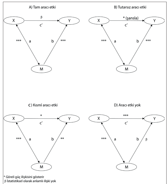
Şekil 2. Aracı etki türleri.
