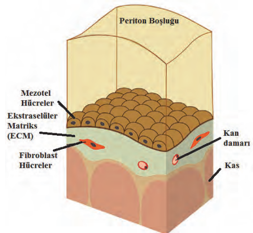
Şekil 3. Peritonun yapısı [17]
