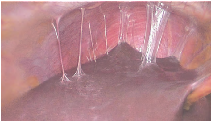
Şekil 4. Gelişmiş adezyon [21]
