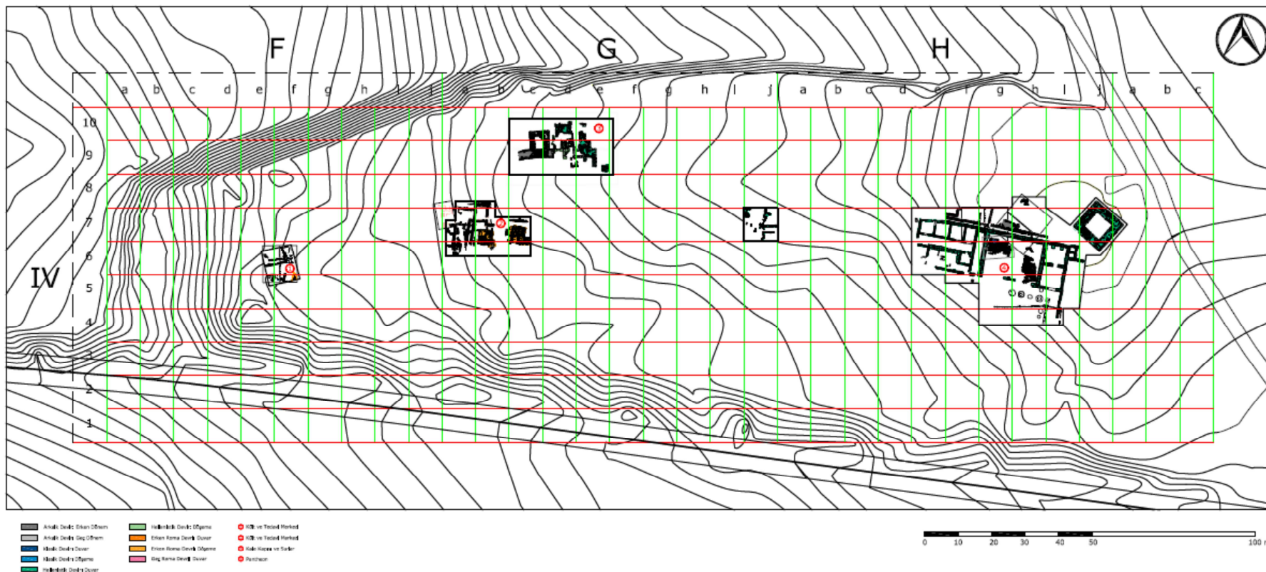
Lev. 2 Heraion Teikhos. Genel Plan.
