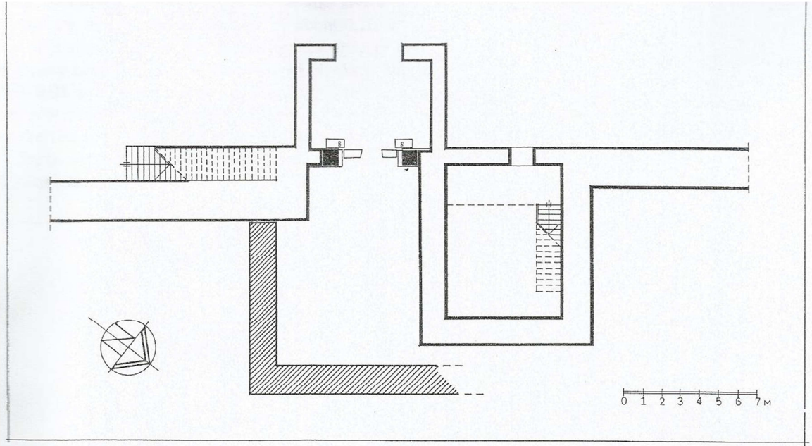
Lev. 12. Kale Kapısı'nın planı (Kolarova 1996: 36)
