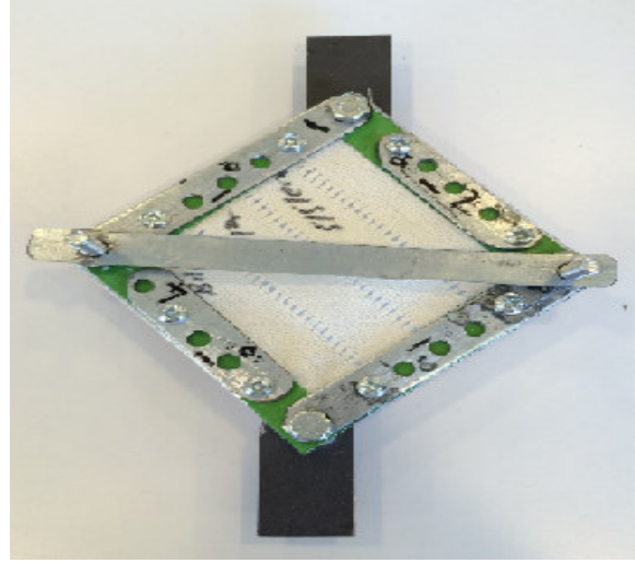
Şekil 3.20. Orta leno/düz çözgü aralığında çerçevenin 90° de başlangıç konumu
