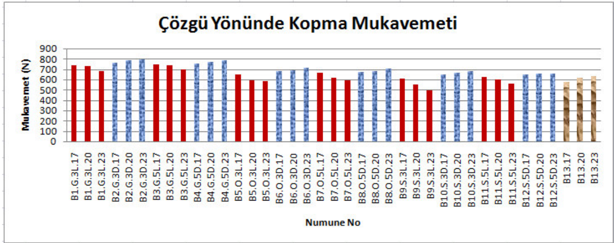
Şekil 4.15. Numunelerin çözgü yönünde ölçülen kopma mukavemeti değerleri (grafikte; kırmızı sütunlar leno bağlantıları, mavi dokulu sütunlar düz bağlantıları, kahverengi dokulu sütunlar ise bezayaği örgüyü gösterir)
