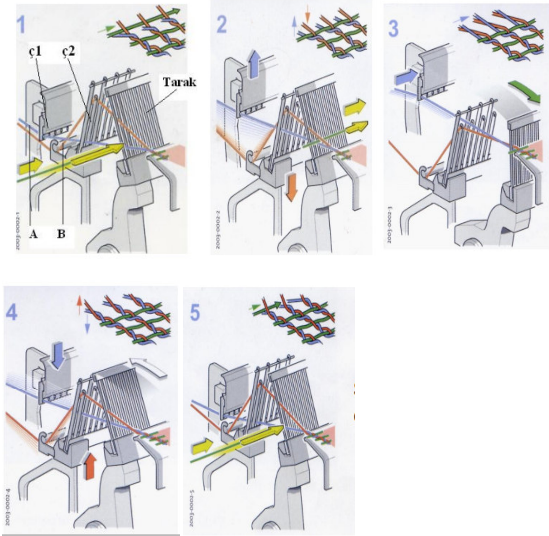
Şekil 2.5. Leno tarak, atkı ve çözümlü hareketi, 1., 2., 3., 4., 5. Pozisyon ( Türkyılmaz 2008)
