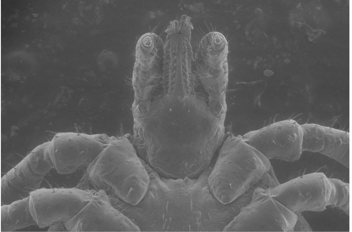
Şekil 4.14. I. kaiseri dişisine ait ağız organellerinin dorsalden ve ventralden (altta) scanning elektron mikroskop görüntüsü.
