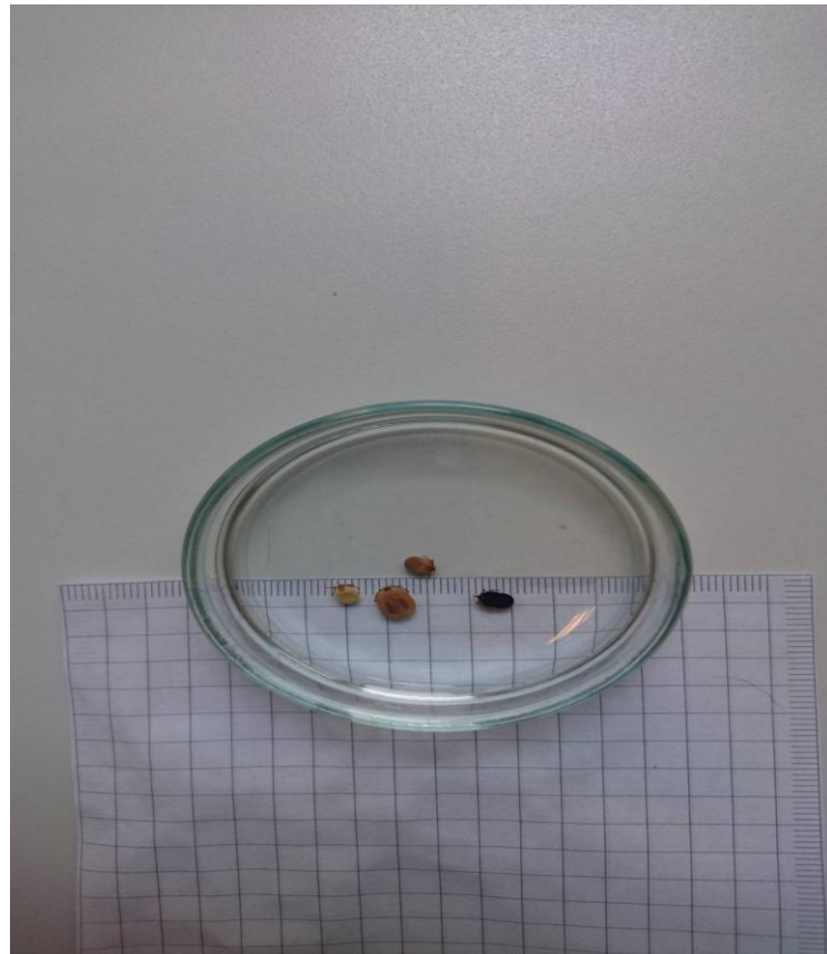
Şekil 4.7. Köpeklerden toplanan I. accuminatus dişisi örnekleri (minimum ölçek 1 mm)
