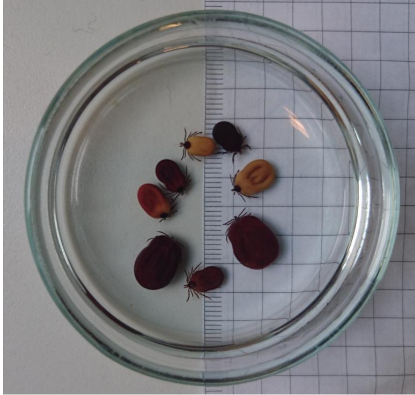
Şekil 4.6. Köpeklerden toplanan I. ricinus dişisi örnekleri (minimum ölçek 1 mm)
