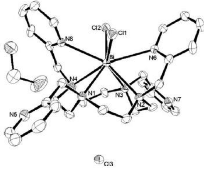
Şekil 4.37. [\text{BiTPCCl}_2]\text{Cl} \cdot 2\text{CH}_2\text{Cl}_2 bileşiğinin kristal yapısı
