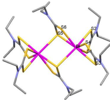
Şekil 4.36. \{[\text{Bi}(\text{Et}_2\text{DTC})_3]_2\} bileşiğinin moleküler yapısı
