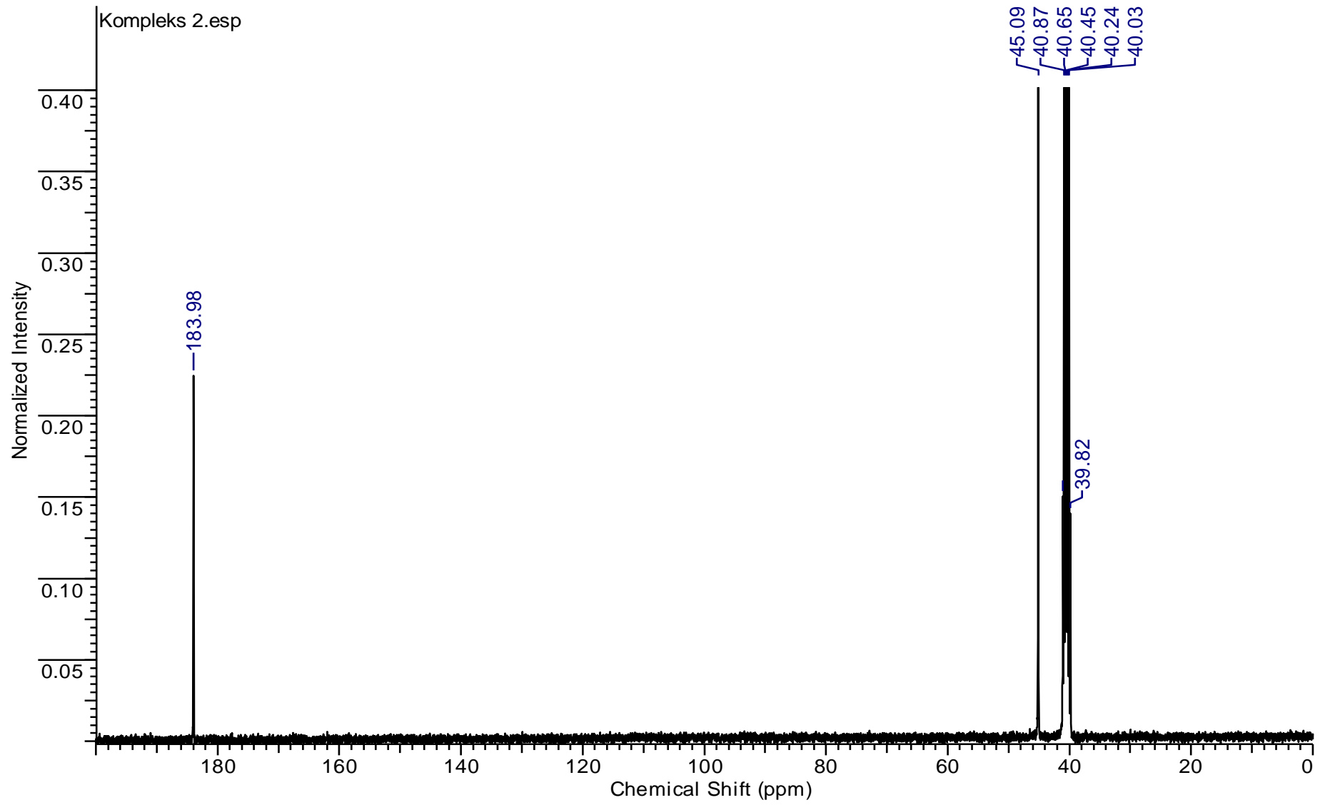
Şekil 9.37. \{[\text{SbBr}_2(\mu_2\text{-Br})(\text{IMT})_2]_2 ( 2 ) bileşiğinin ^{13}\text{C} -NMR spektrumu
