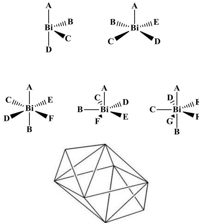
Şekil 4.24. Bizmut(III) bileşiklerinin olası geometrileri
