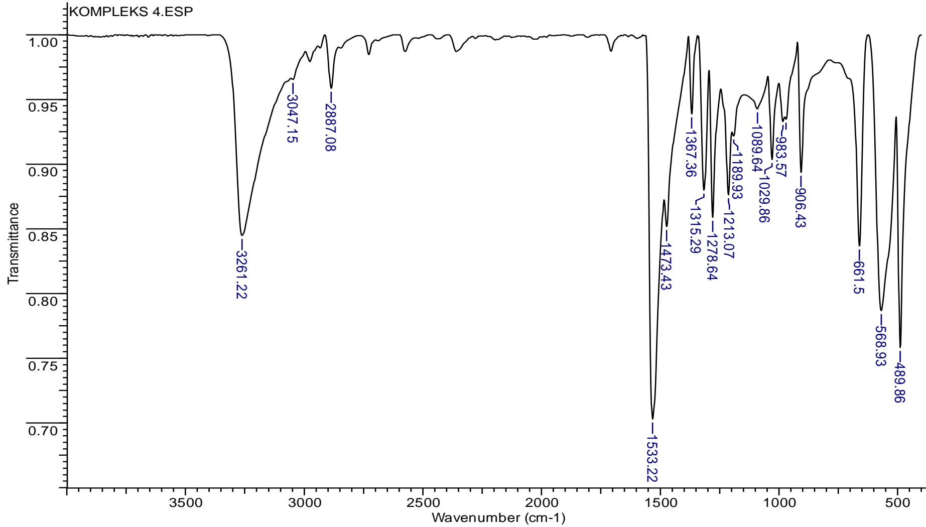
Şekil 9.9. [\text{BiCl}_3(\text{IMT})_2] (4) bileşiğinin infrared spektrumu
