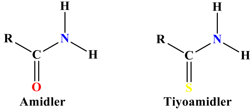
Şekil 6.1 Amidler ve tiyoamidlerin genel formülleri
