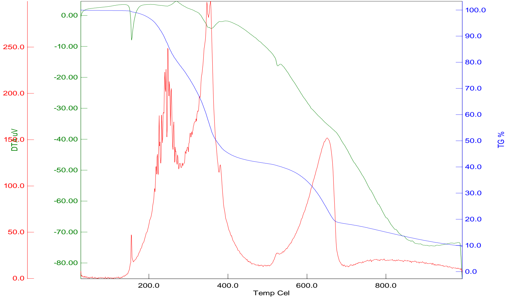
Şekil 9.22. [SbCl_2(\mu_2-Cl)(IMT)_2]_2 (1) bileşiğinin TG-DTA eğrisi
