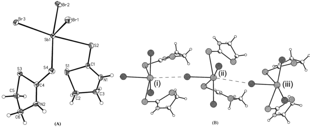
Şekil 4.12. \{[\text{SbBr}_2(\mu_2\text{-Br})(\text{MTZD})]_n\} bileşiğinin monomer ve polimer yapısı
