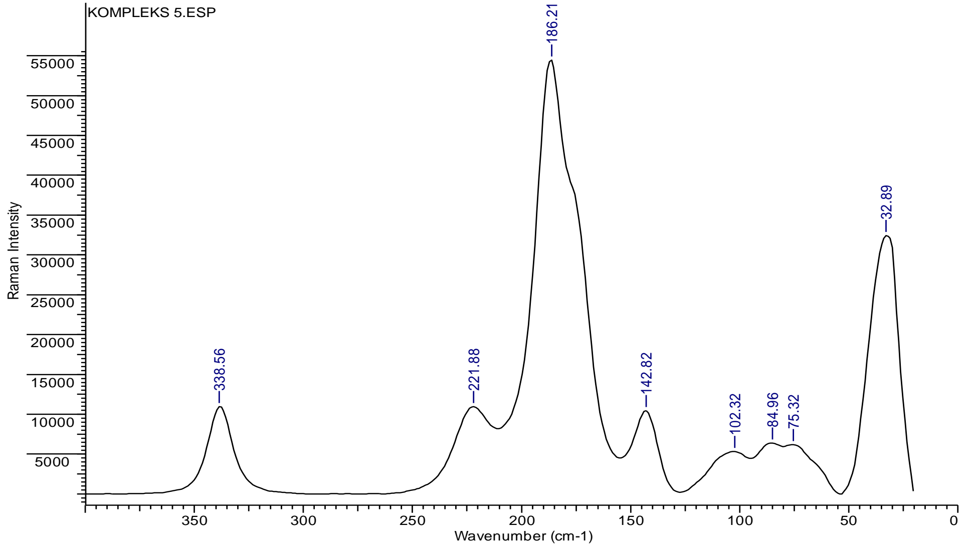
Şekil 9.18. [\text{BiBr}_3(\text{IMT})_2] (5) bileşiğinin raman spektrumu
