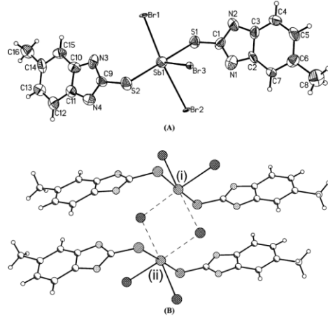
Şekil 4.14. \{[SbBr_2(\mu_2-Br)(MMBZIM)_2]_2\} bileşiğinin monomer ve polimer yapıları
