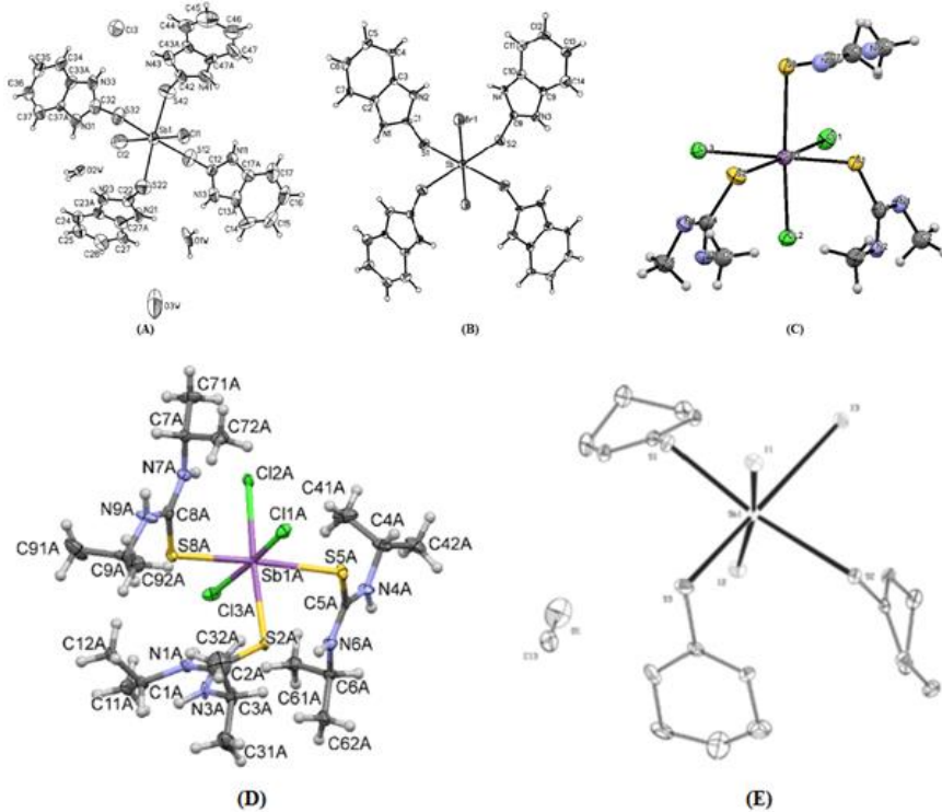
Şekil 4.22. \{[SbCl_2(MBZIM)_4]^+ \cdot Cl^- \cdot 3H_2O \cdot (CH_3CN)}\} (A), \{[SbBr_2(MBZIM)_4]^+ [Br]^- (H_2O)}\} (B), fac- [SbCl_3(DMTU)_3] (C), mer- [SbCl_3(DIPTU)_3] (D) ve \{[SbI_3(tHPMT)_3] \cdot MeOH}\} (E) bileşiklerinin kristal yapıları
