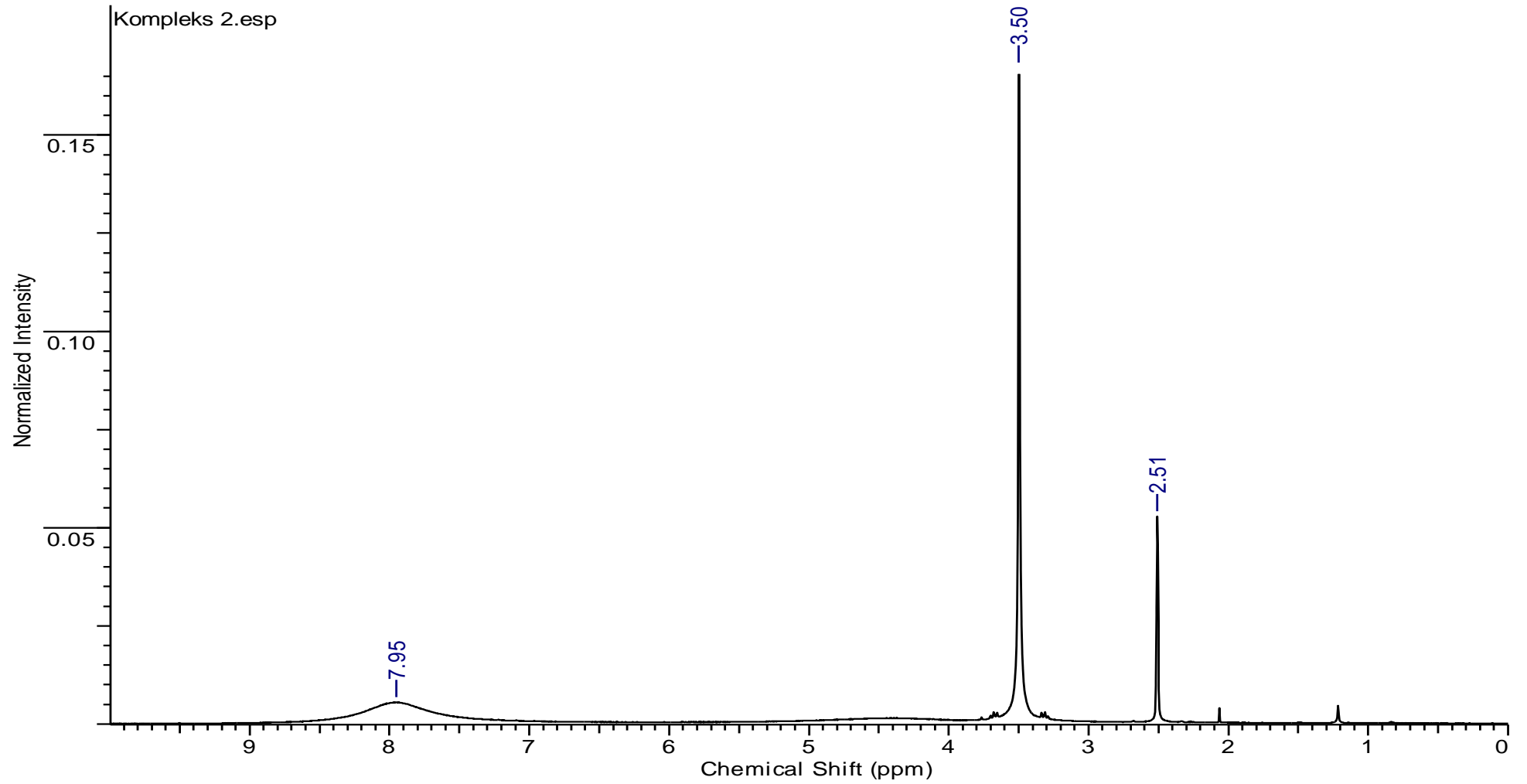
Şekil 9.30. [\text{SbBr}_2(\mu_2\text{-Br})(\text{IMT})_2]_2 ( 2 ) bileşiğinin ^1\text{H-NMR} spektrumu
