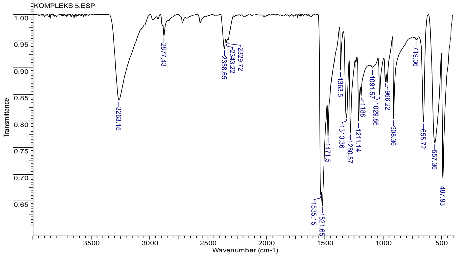
Şekil 9.10. [\text{BiBr}_3(\text{IMT})_2] (5) bileşiğinin infrared spektrumu
