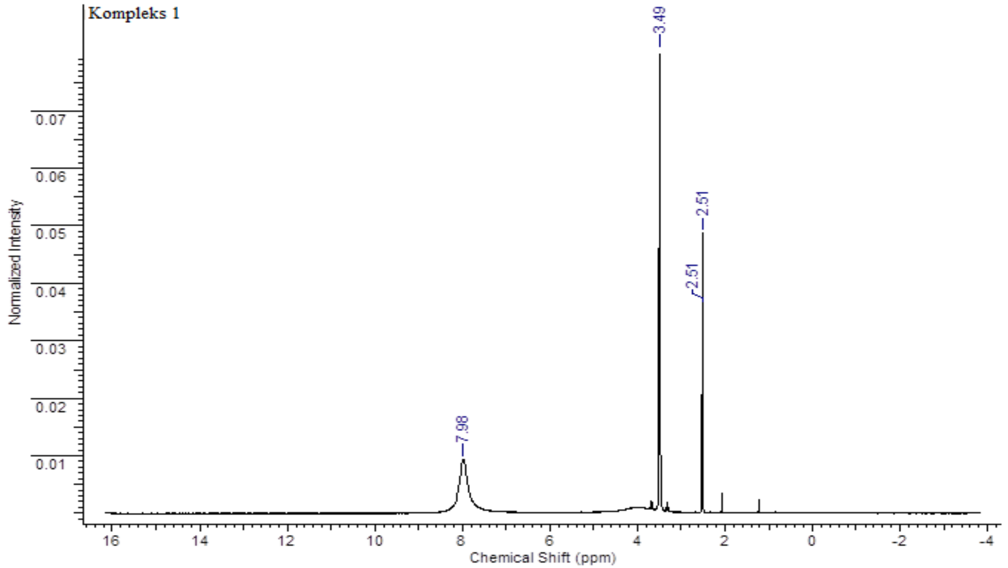
Şekil 9.29. \{[\text{SbCl}_2(\mu_2\text{-Cl})(\text{IMT})_2]_2 ( 1 ) bileşiminin ^1\text{H-NMR} spektrumu
