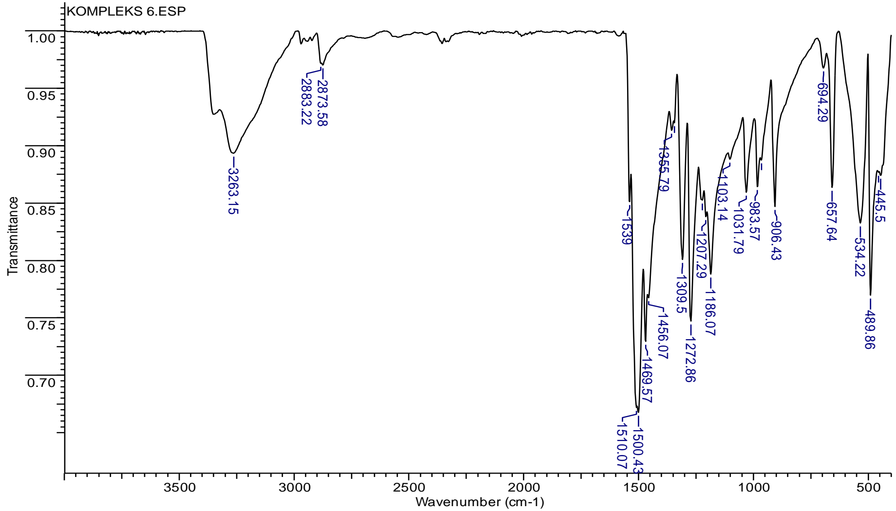
Şekil 9.11. [\text{BiI}_3(\text{IMT})] (6) bileşiğinin infrared spektrumu
