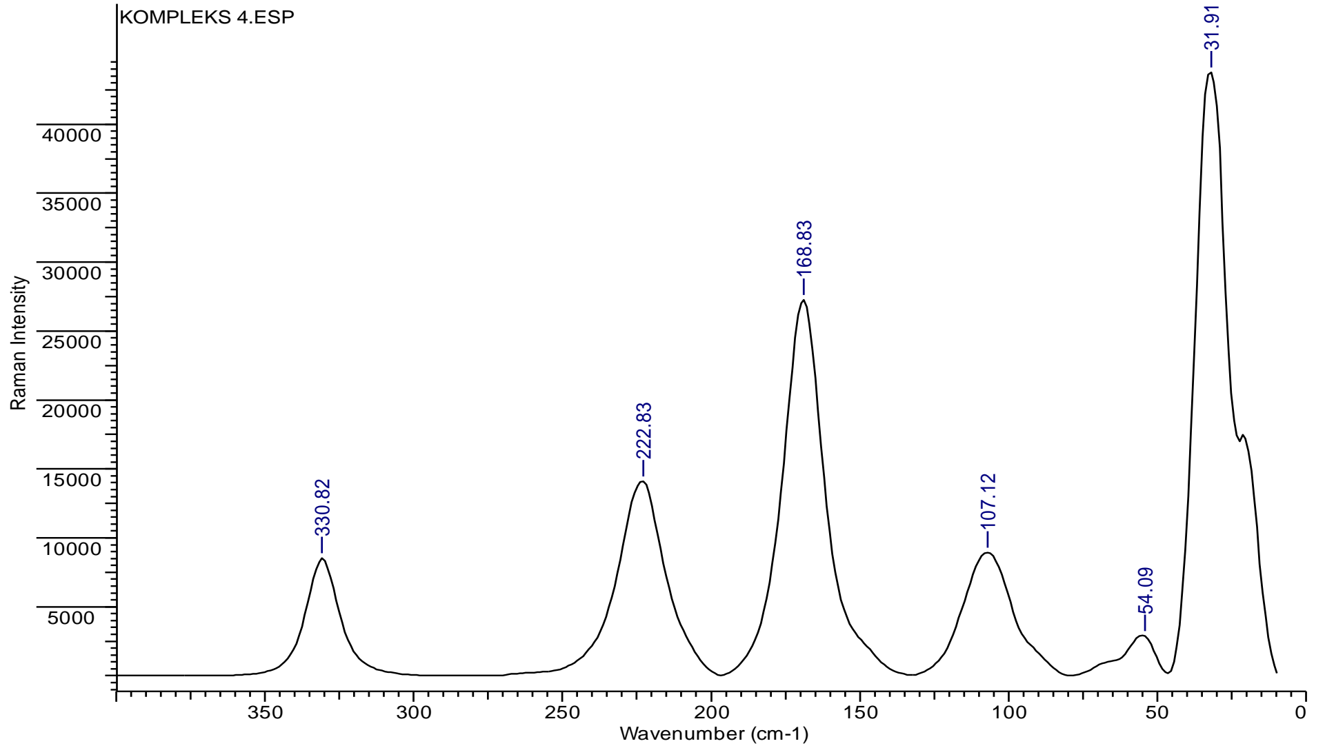
Şekil 9.17. [BiCl 3 (NT) 2 ] (4) bileşiğinin raman spektrumu
