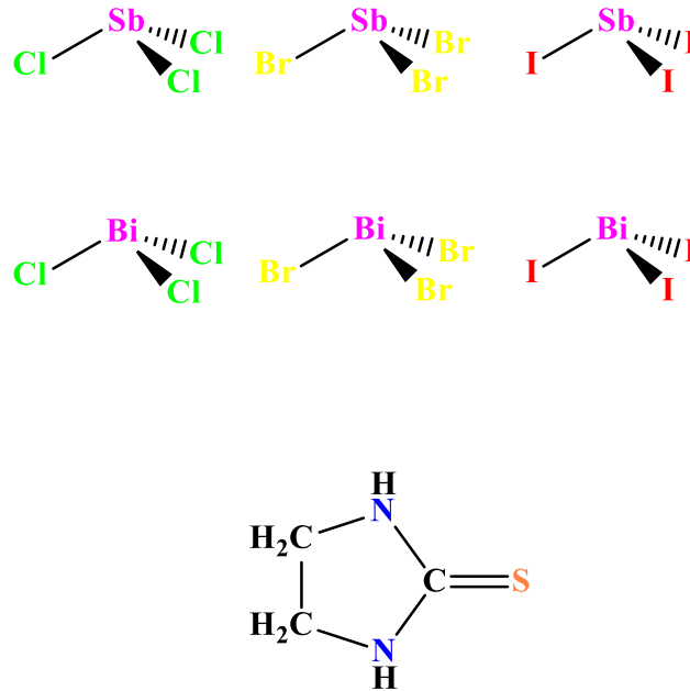
Şekil 9.1 Kullanılan VA grubu halojenürlerin ve 2-imidazolidintiyonun kimyasal yapıları
