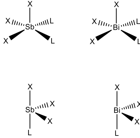
Şekil 9.4. Sentezlenen bileşiklerin geometriler
