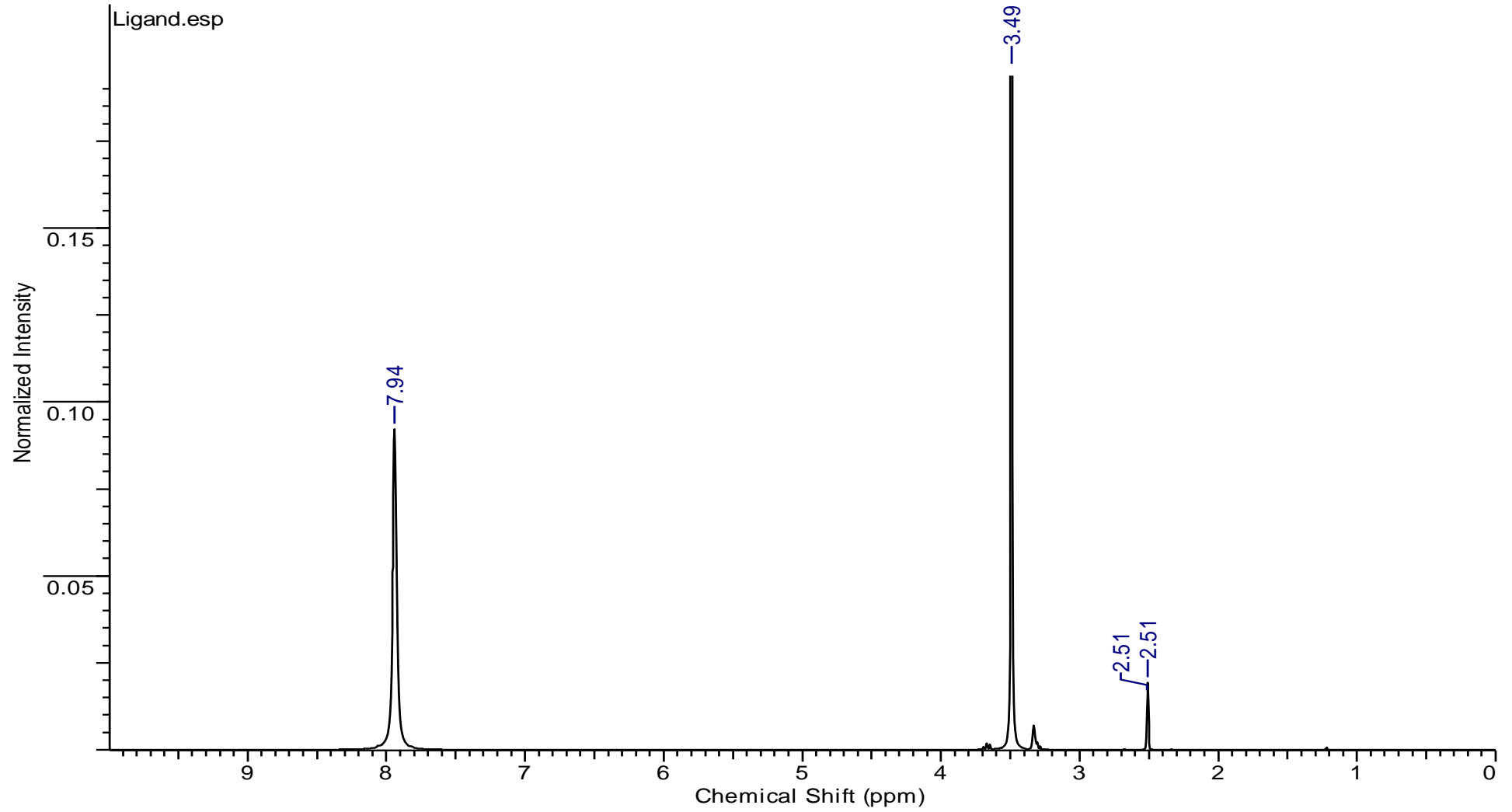
Şekil 9.28. 2-İmidazolidintiyonun ^1\text{H} -NMR spektrumu
