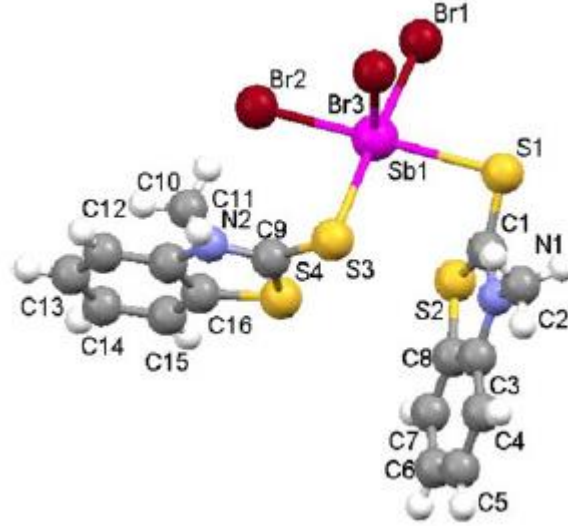
Şekil 4.11. [\text{SbBr}_3(\text{MMBZT})_2] bileşiğinin kristal yapısı
