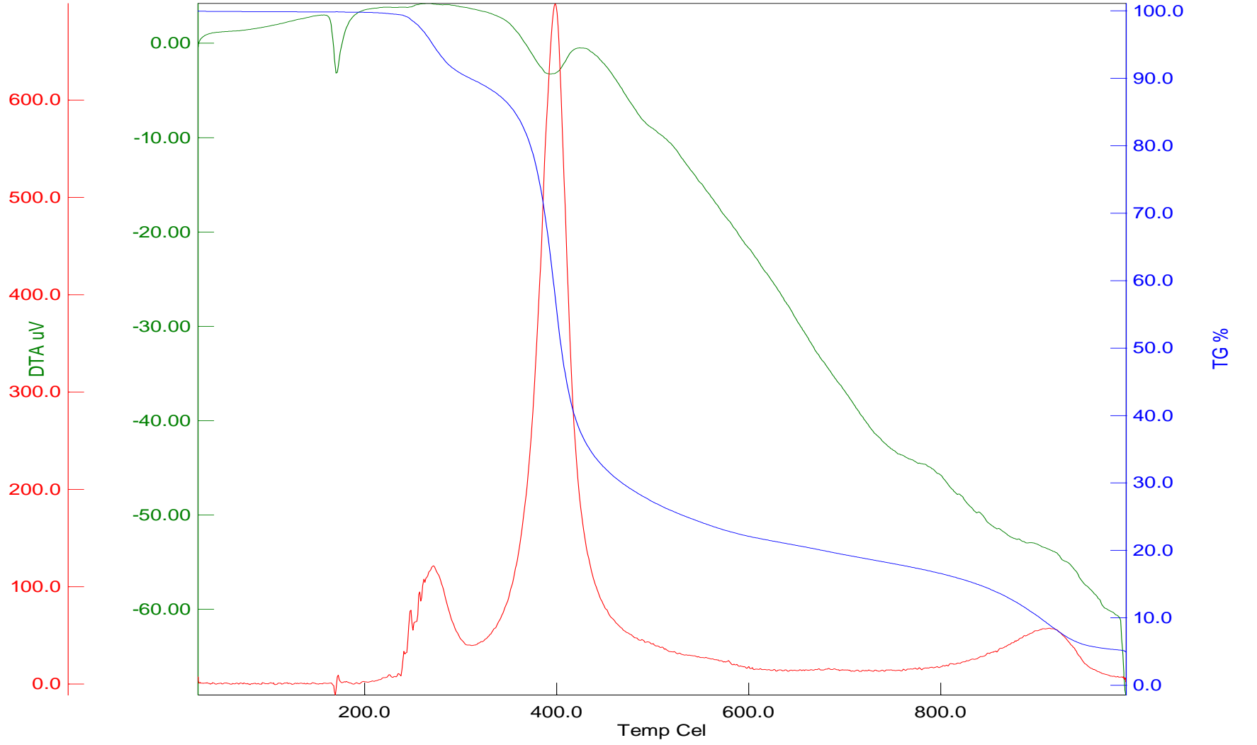
Şekil 9.26. [\text{BiBr}_2(\mu_2\text{-Br})(\text{IMT})_2]_2 (5) bileşiğinin TG-DTA eğrisi
