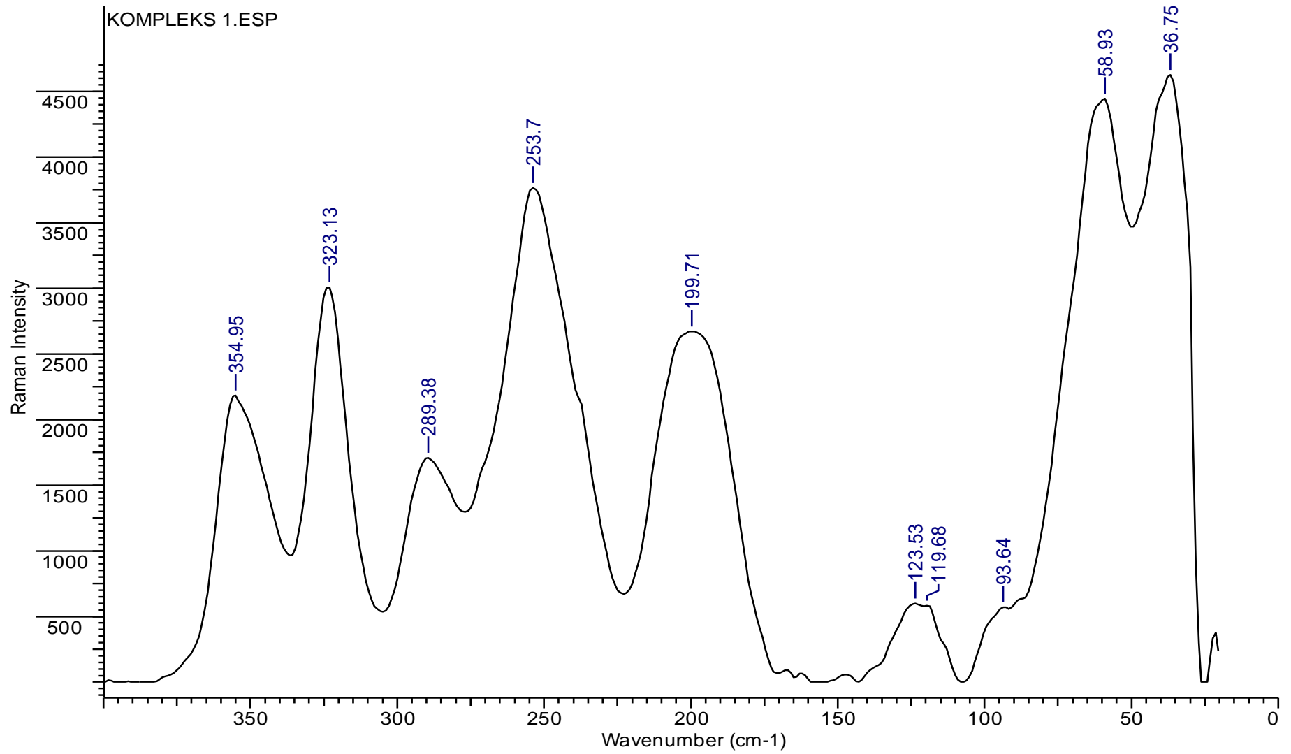
Şekil 9.14. [\text{SbCl}_3(\text{IMT})_2] (1) bileşiğinin raman spektrumu
