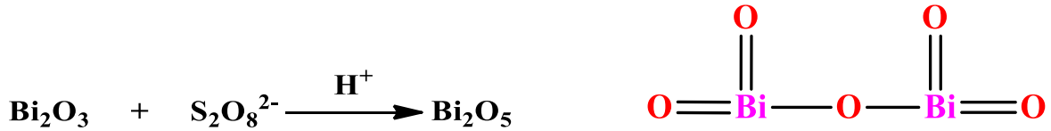
Şekil 3.5. Bizmut (V) oksidin oluşum reaksiyonu ve molekül yapısı
