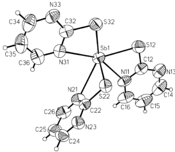
Şekil 4.23. [\text{Sb}(\text{PMT})_3] \cdot 0.5(\text{CH}_3\text{OH}) bileşiğinin kristal yapısı
