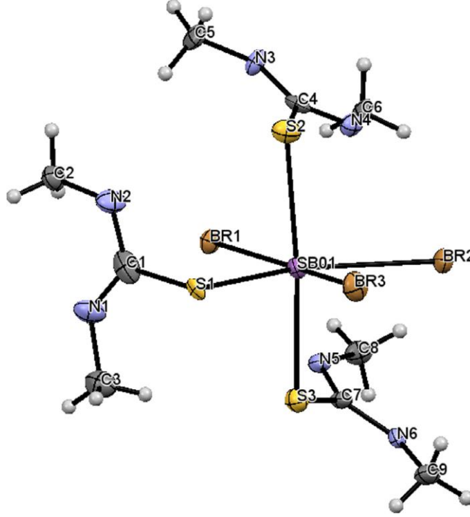
Şekil 4.20. [SbBr_3(DMTU)_3] bileşiğinin kristal yapısı
