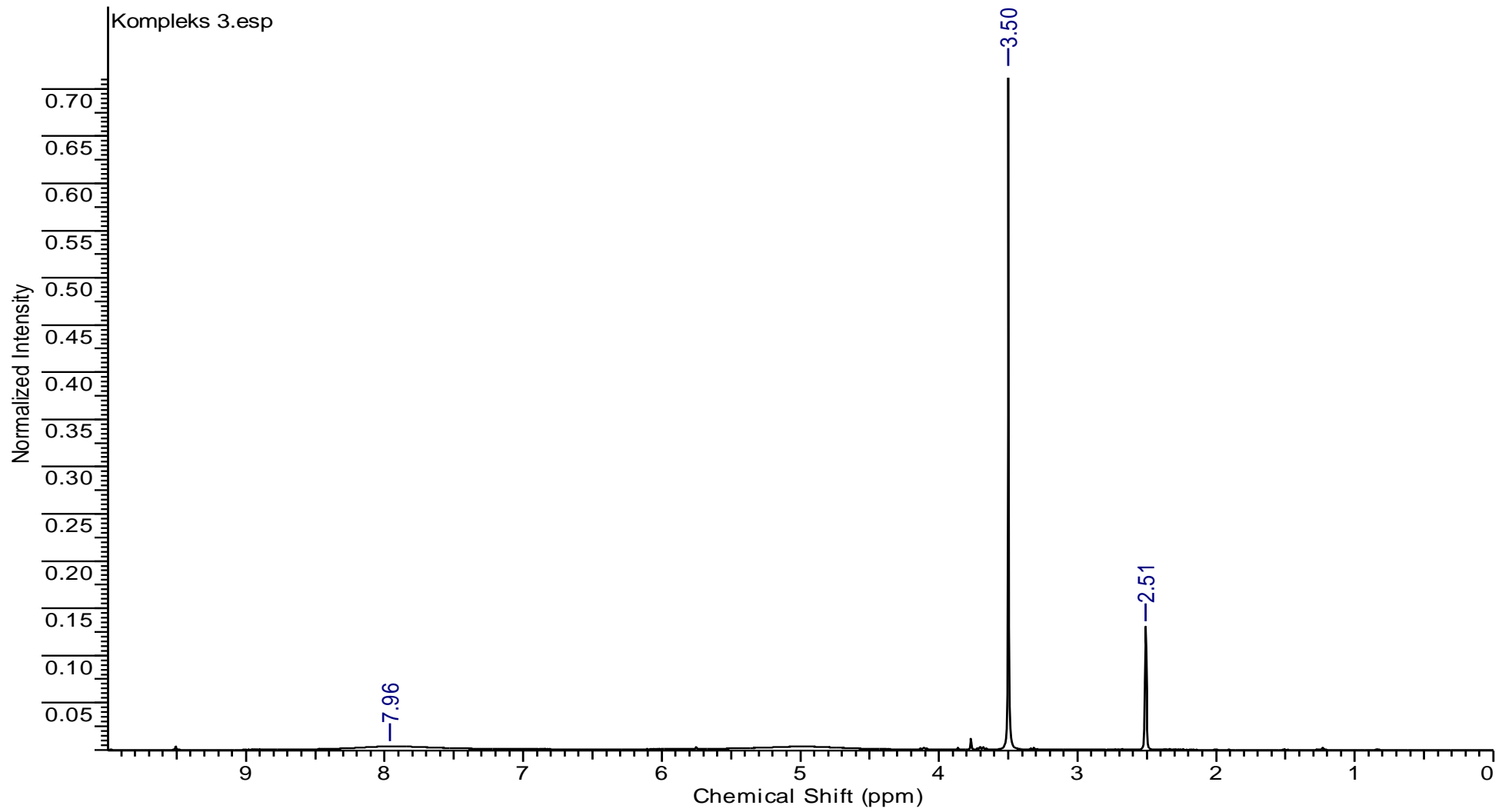
Şekil 9.31. \{[\text{SbI}_2(\mu_2\text{-I})(\text{IMT})]_n\} ( 3 ) bileşiğinin ^1\text{H-NMR} spektrumu
