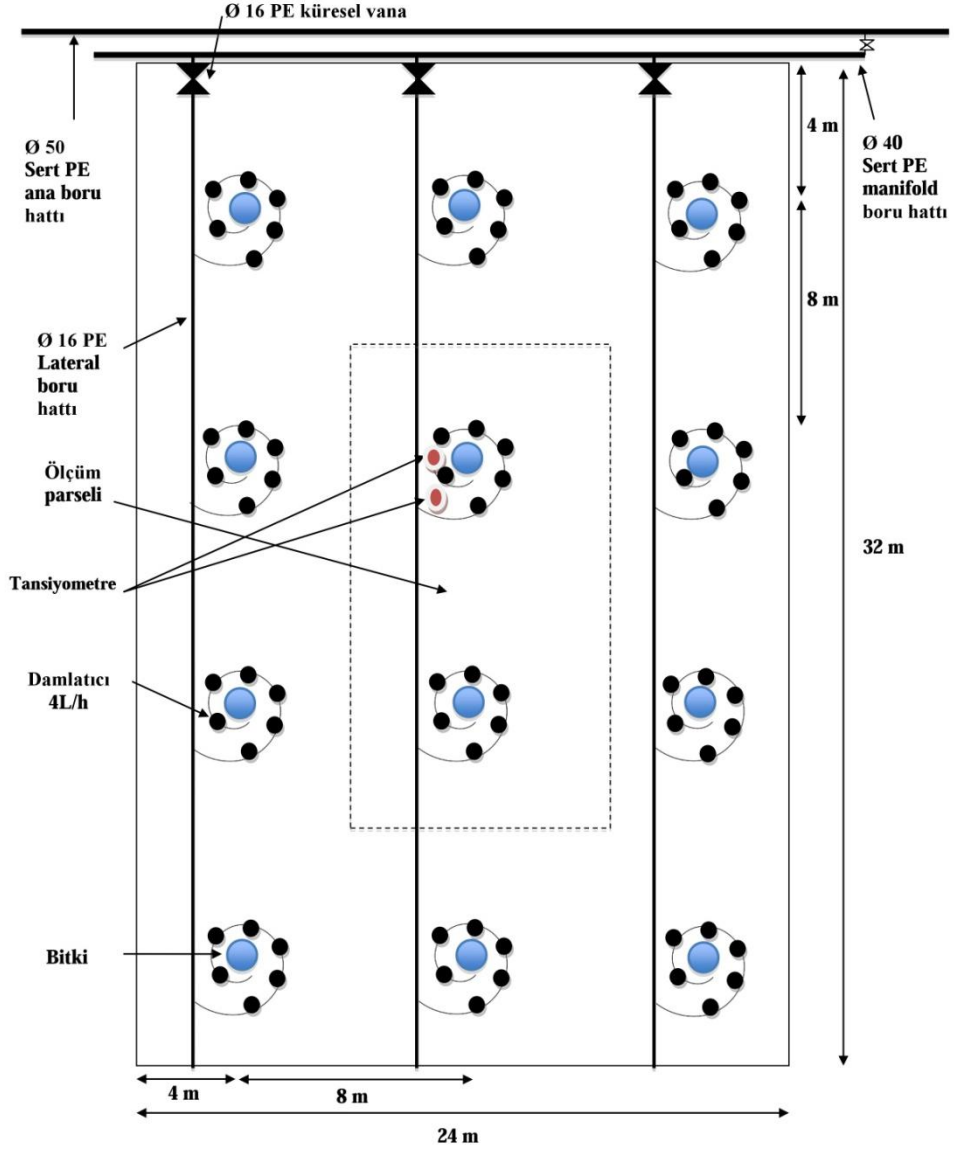
Şekil 3.5. Deneme alanında kurulan salkım tertip damla sulama sistemi
