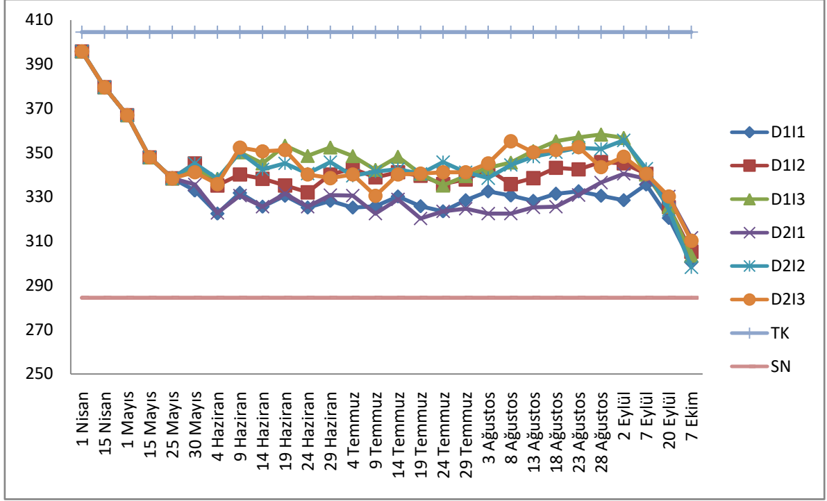
Şekil 4.5. Bitki gelişim periyodu boyunca sulama öncesi topraktaki nem değışimleri, (2016 yılı)
