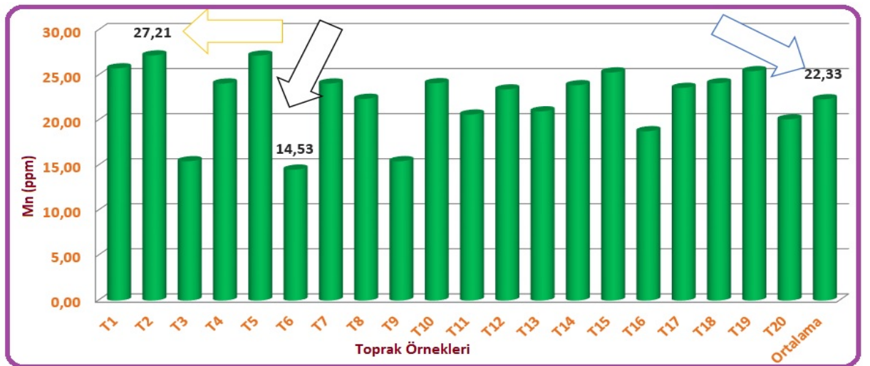
Şekil 4.10. Toprak örneklerindeki Mn değerleri ( \text{mg kg}^{-1} ) (ppm)
