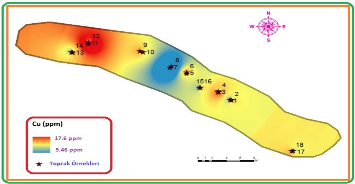
Şekil 4.40. Bakır elementi mekânsal dağılım haritası
