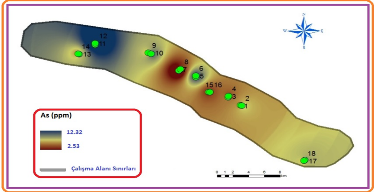
Şekil 4.45. Arsenik elementi mekânsal dağılım haritası
