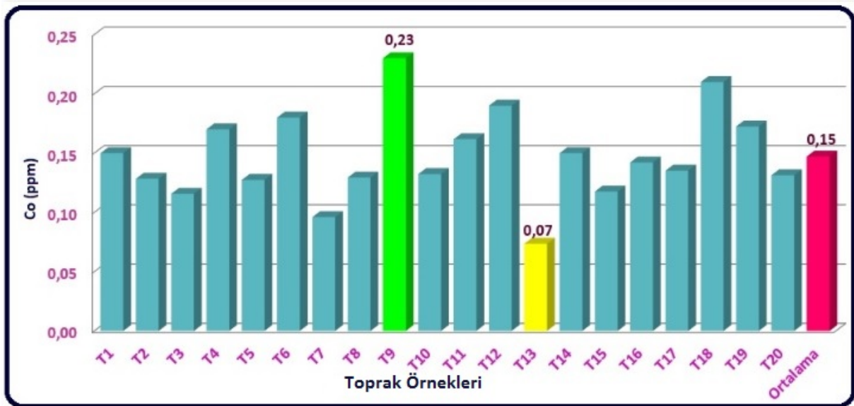
Şekil 4.5. Toprak örneklerindeki Co değerleri ( \text{mg kg}^{-1} ) (ppm)
