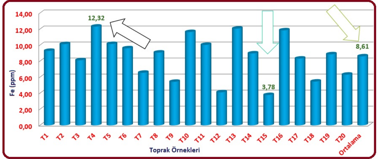
Şekil 4.9. Toprak örneklerindeki Fe değerleri ( \text{mg kg}^{-1} ) (ppm)
