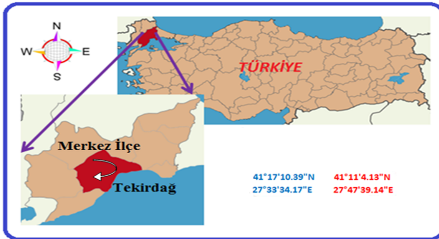
Şekil 3.1. Araştırmanın yapıldığı Tekirdağ ilinin yeri ve konumu (orijinal)
