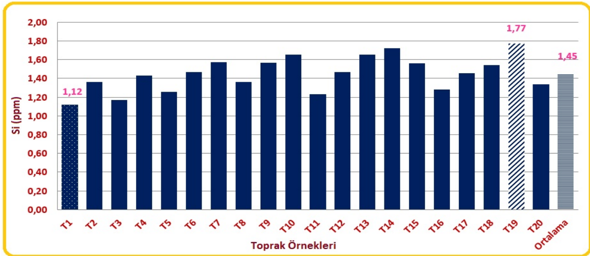
Şekil 4.15. Toprak örneklerindeki Si değerleri ( \text{mg kg}^{-1} ) (ppm)
